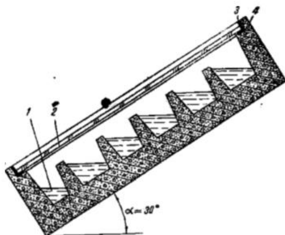
Рис. 2. Схема элемента солнечного опреснителя наклонно-ступенчатого типа.
