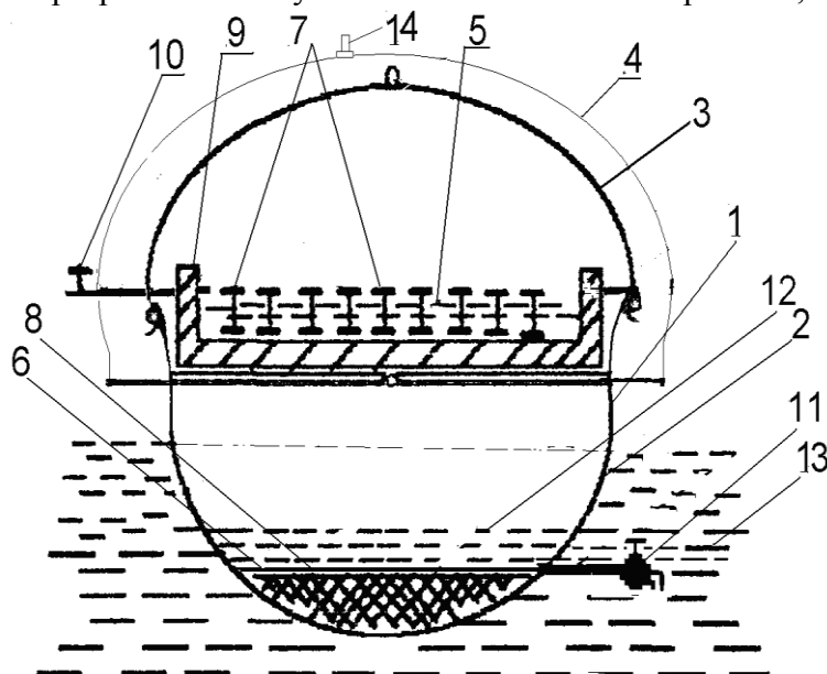
Рис. 3. Устройство плавучего солнечного опреснителя сН-образного металлического теплоприемника
