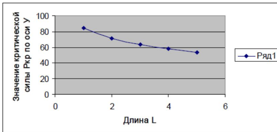
Рис.3.График зависимости значений критической силы от изменений пролета по оси Y
