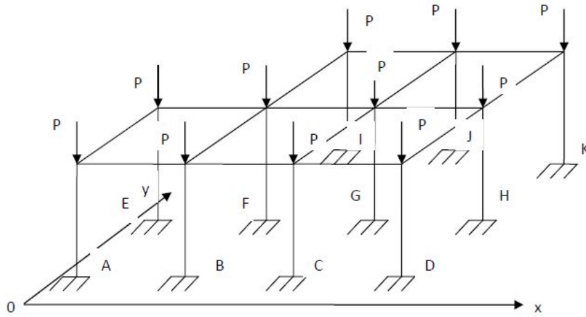
Рис.2.Пространственный рамный каркас
