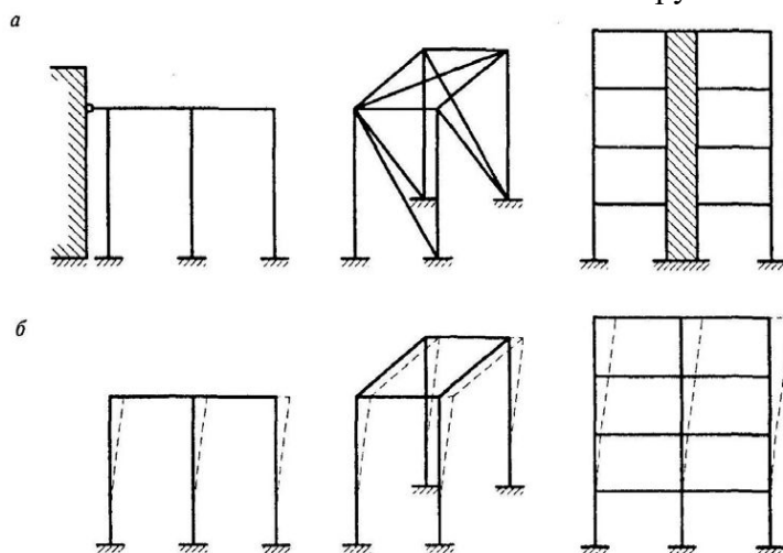
Рис.1. Схемы систем раскрепленных (а) и не раскрепленных от перемещений (б)
