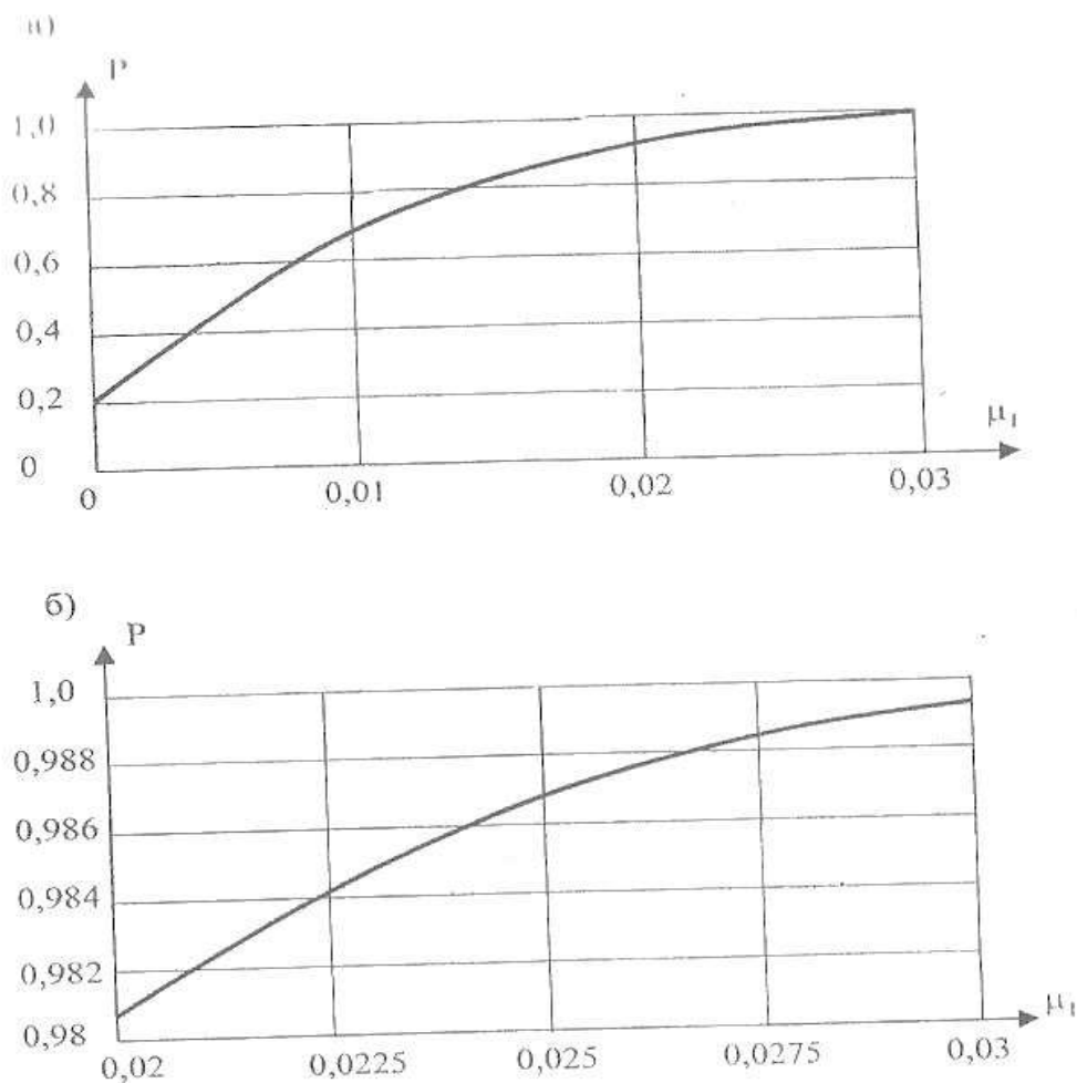
Рис.4. График зависимости обеспеченности несущей способности N=1718,25 \text{ кН} от коэффициента армирования \mu_1
