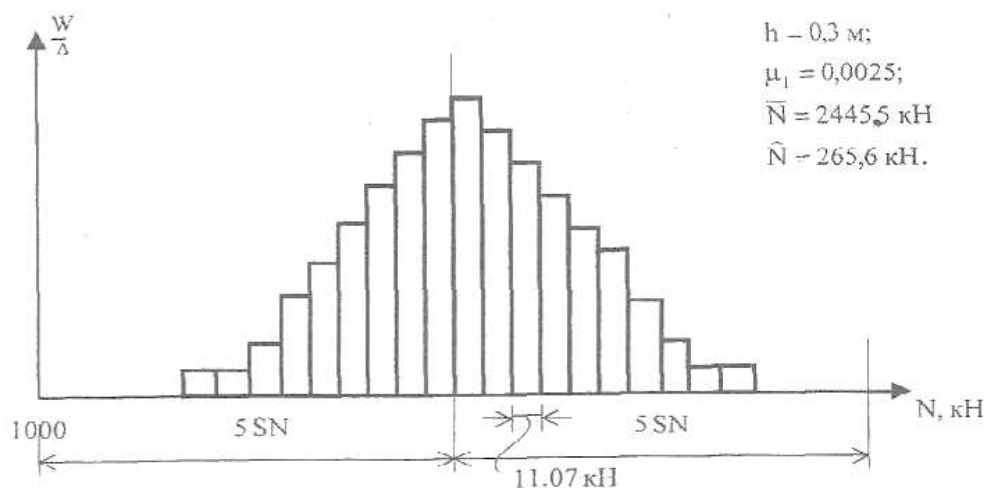
Рис.2. Гистограмма относительных частот функций распределение несущей способности железобетонного стержня, отнесенных к числу интервалов разбиение
