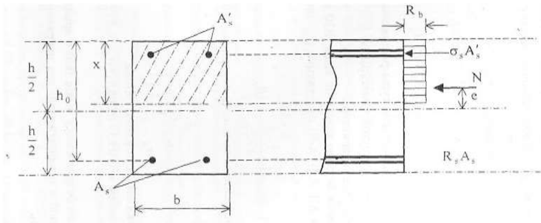
Рис.1. Расчетная схема сечения железобетонного элемента
