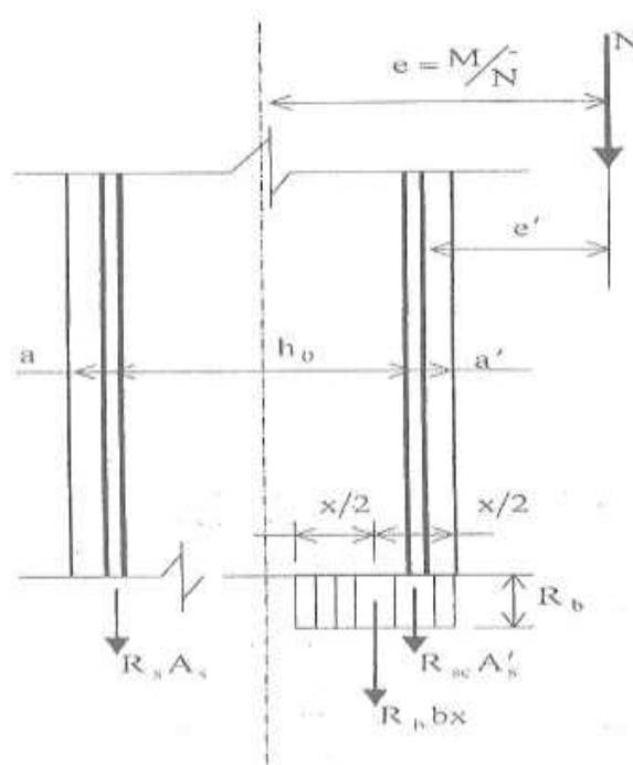
Рис.5. Расчетная схема внецентренного сжатого элемента
