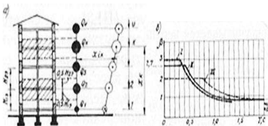
Рис.1. Схемы к определению на здание сейсмических нагрузок.
